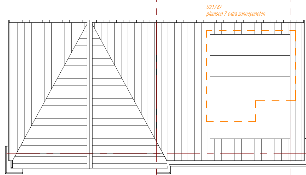
dakaanzicht 1 : 100
