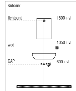
aanzicht wastafel badkamer elektra hoogte
